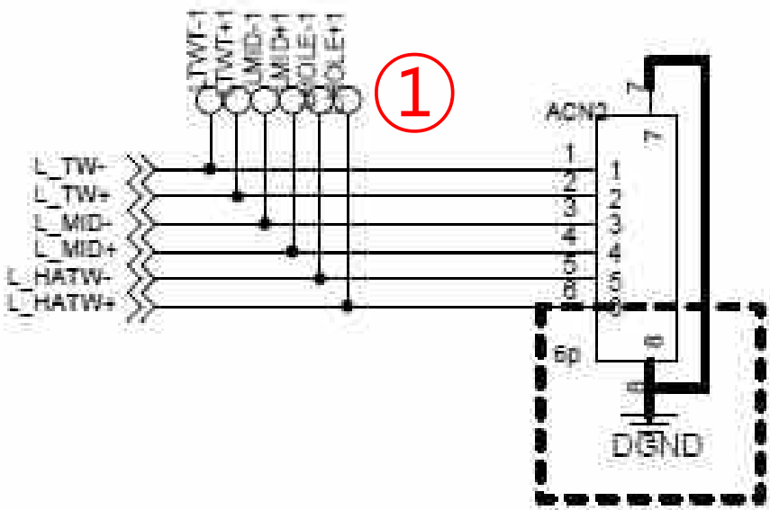
LEFT 3 SPK.
